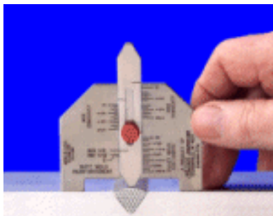
Comprobación sobre- espesor soldadura a tope
